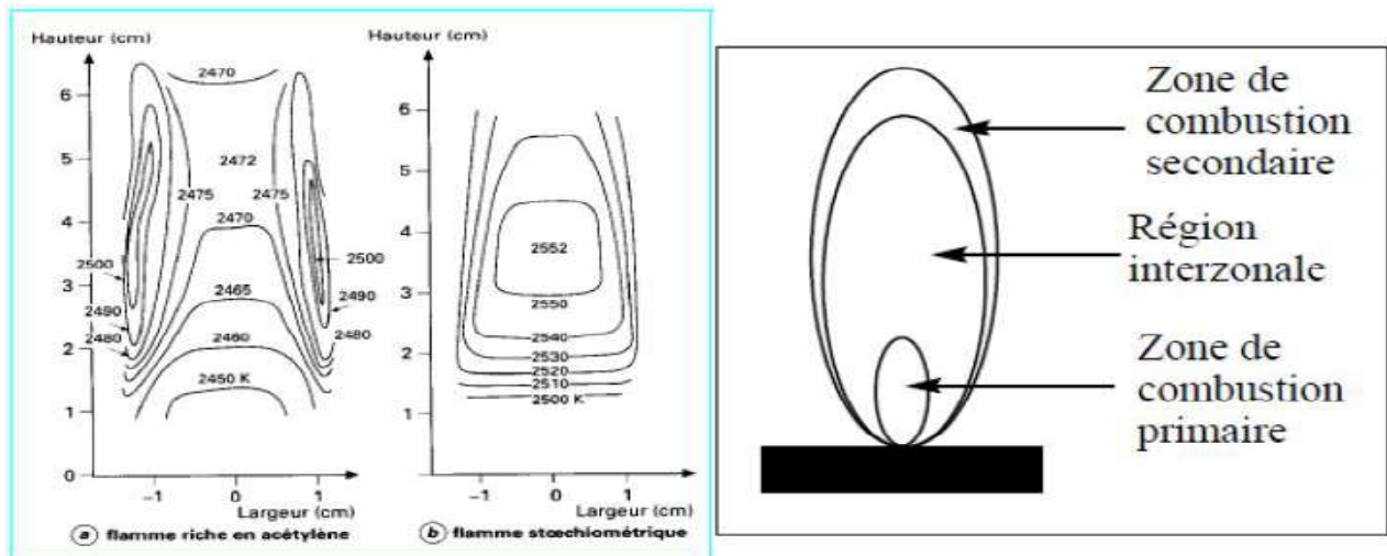
Figure 8 : profil de température dans une flamme air-acétylène
