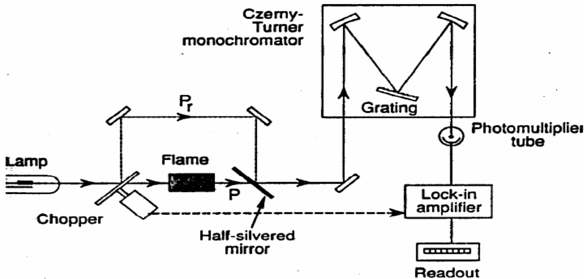
Figure 4 : Schéma du spectromètre à deux faisceaux.
