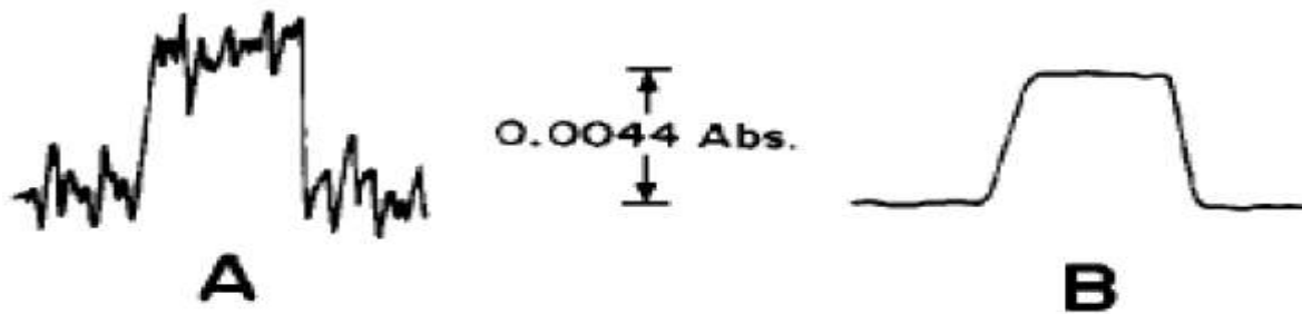
Figure 14 : Deux situations différentes avec la même sensibilité et des limites de détection différente. Il est clair que dans le cas B ,On distingue de plus petites variations d'absorbance que dans le cas A ,Ou le signal est plus bruité.
