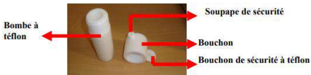
Figure 13 : Système de minéralisation utilisant une bombe à téflon.
