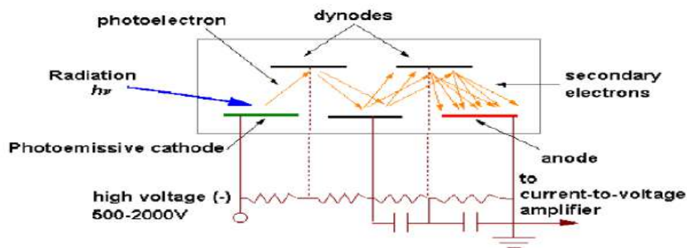
Figure 12 : Principe de tube multiplicateur
