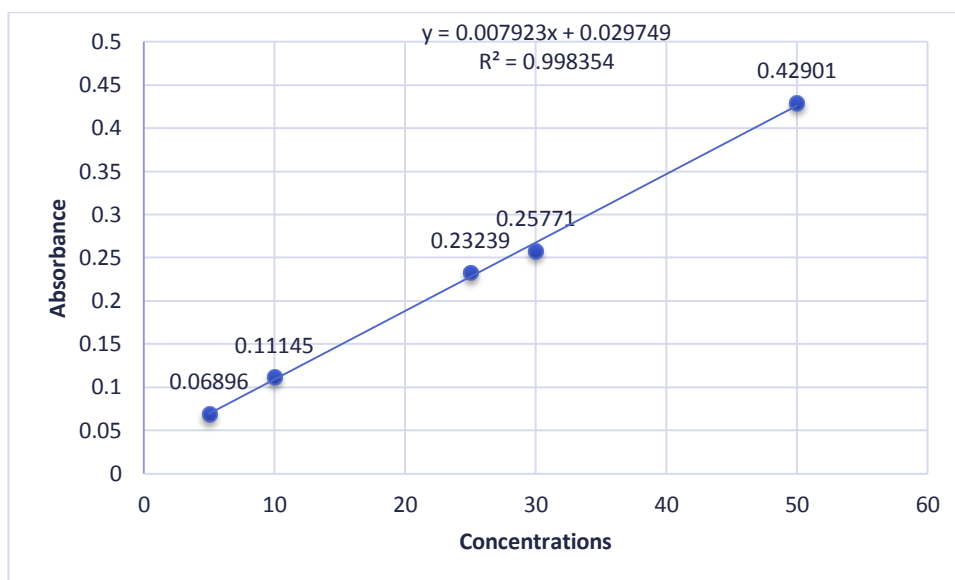
Figure 17 : Courbe d'étalonnage (concentration en plomb en fonction de l'absorbance).
